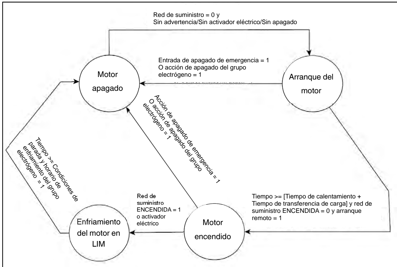
Figura 6: Modo SMD para AMF
