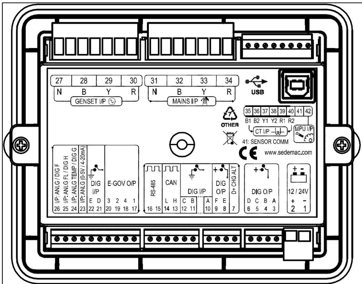
Figure 1 : Contrôleur du groupe électrogène GC1031 depuis l'arrière
