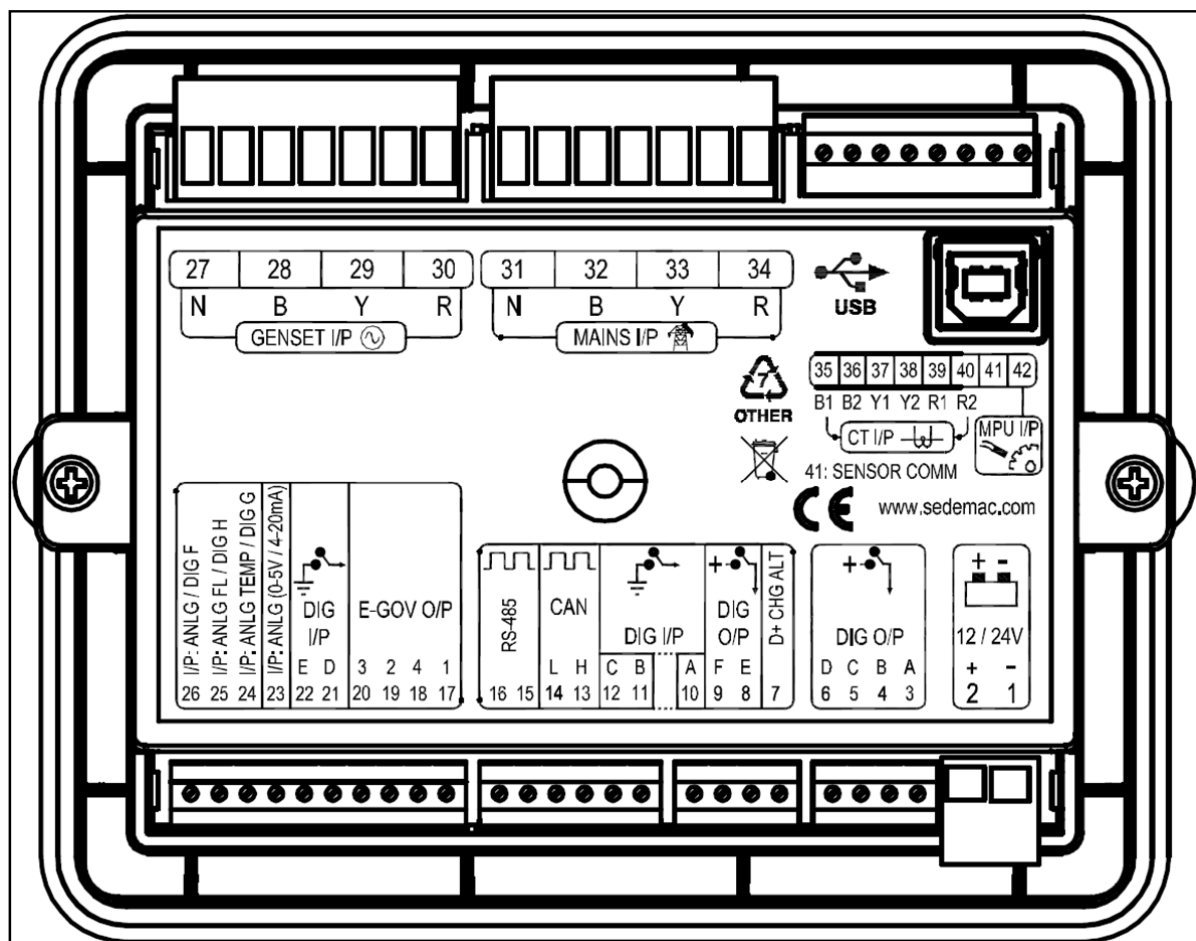
Figura 1: Vista posterior del controlador de grupo electrógeno GC1031
