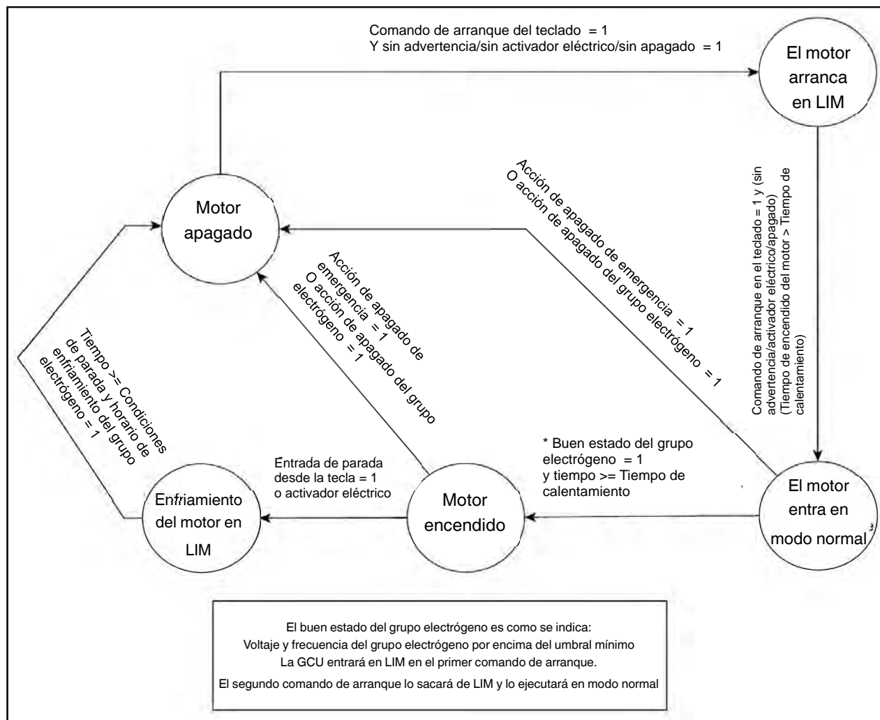
Figura 8: SMD para modo manual
