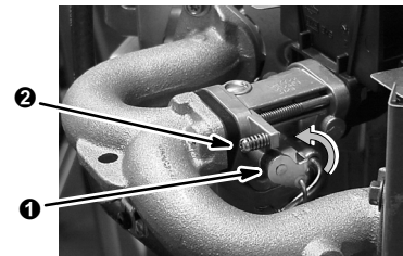
Single Barrel De Un Solo Cuerpo Simple corps
